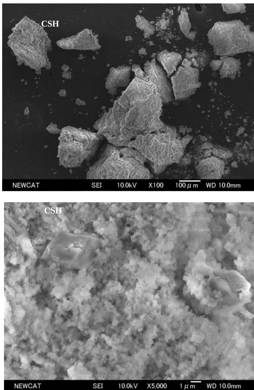
写真1 メタケイ酸ナトリウムと塩化カルシウムから生成した CSH の走査型電子顕微鏡写真
